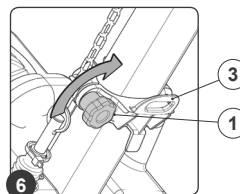
7. Inserire la catenella tirante rubinetto serbatoio soluzione (6) nel gancio presente nella maniglia comando rubinetto (7) (Fig.8).
